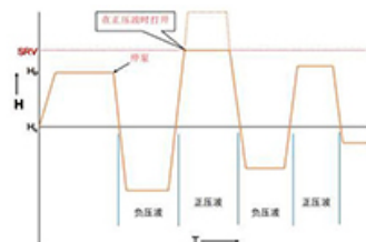
安装水击泄放阀后
