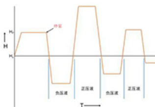
未装水击泄放阀
